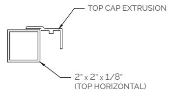
TOP CAP
